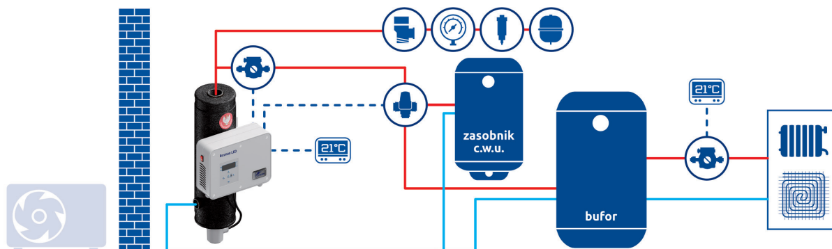
Wariant 2: jako urządzenie samodzielne w oczekiwaniu na montaż pompy ciepła lub innego źródła ciepła
