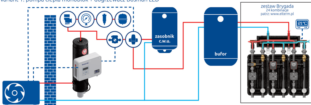
Wariant 1: pompa ciepła monoblok + dogrzewacz Bosman LED
