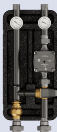
Zawór mieszający ESBE VTA 322
