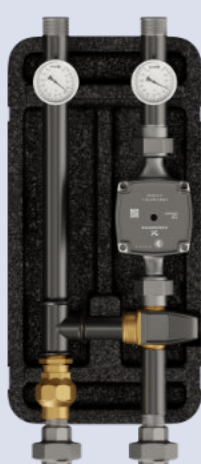
Zawór mieszający ESBE VTA 522
