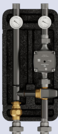
Zawór mieszający termostatyczny ESBE VTA 322
